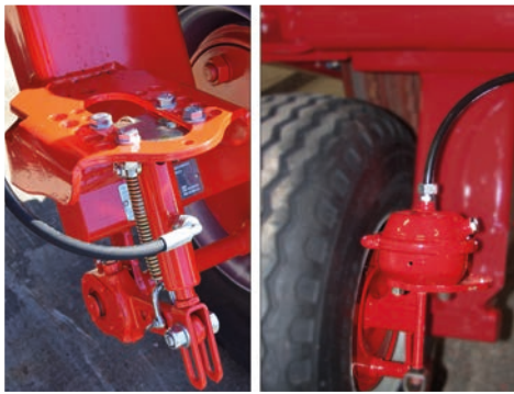
Hydrauliske / Tryklufsbremser
