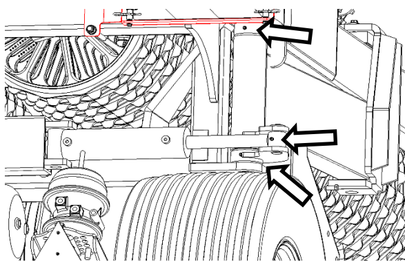
1 nippel på foldecylinder og 2 stk. på vingenagle 10 timer
