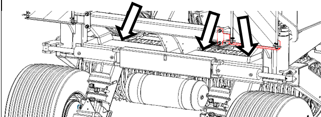
3 nipler på hængselled mellem bagstjært og hjulstel 30 timer
