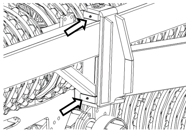
2 nipler på vingers vippeled 10 timer
