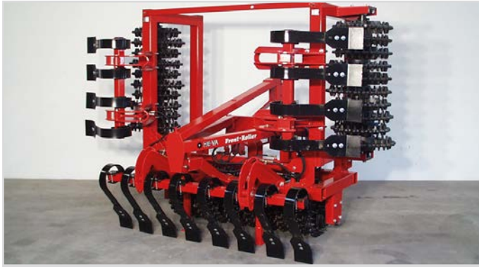
4,00 m Front-Roller m/ Crosskill, hydr. Klappung und Spring-Board.
