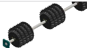
Rouleau étoile Ø450/Ø500 mm - (synchronisé - 400 mm en largeur à l'arrière de chaque dent)
