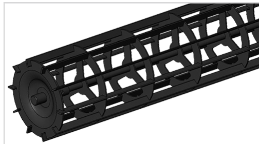
Flachstabwalze Ø410 mm
