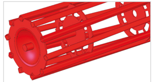
Rohrstabwalze Ø550 mm
