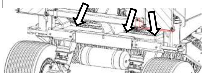
3 Nippel am Drehgelenk zwischen hinterer Deichsel und Radrahmen 30 Stunde
