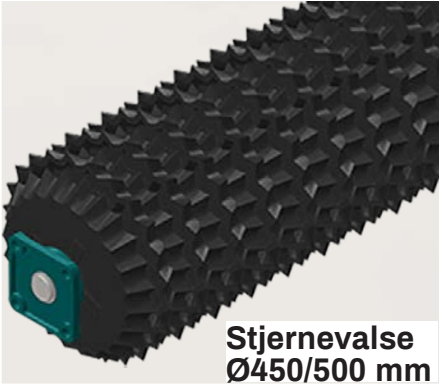
Svær rørvalse Ø500 mm
