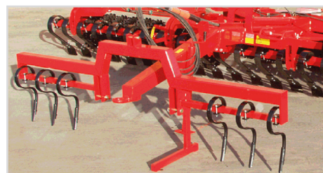
Spårluckringssats, trepunktupphängd
