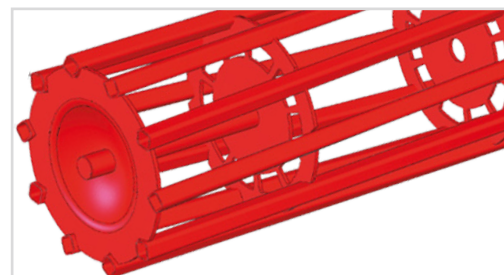
Rörvals Ø550 mm
