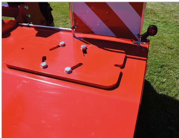
Ekstra vægte á 30 kg. Max 90 kg./m
