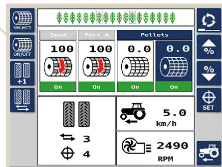
Exemple: Interface HE-VA ISOBUS sur Terminal Topgun
