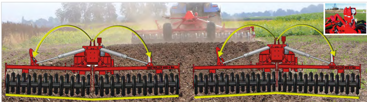
Standardutrustning på 2- och 3-sektion modeller: HE-VA SAT-System: Hydr. justerbar viktöverföringssystem, som säkrar en jämn vikt-överföring på hela arbetsbredden och som samtidigt påverkar att sidosektionerna följer marken.
