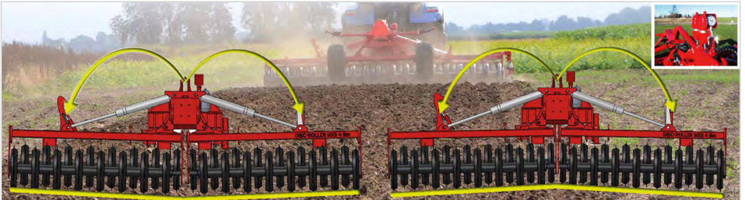
Standardudstyr på 2- og 3-leds modeller: HE-VA SAT-System: Hydraulisk justerbar vægtoverføringsystem, der sikrer ens vægtoverføring i hele arbejdsbredden og samtidig bevirker at vingesektionerne følger terrænet.
