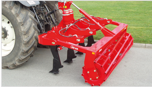
3,00 m m/hydraulisk stenutlösning, 4 pinnar, rörvals med fyrkantsrör och hydr.djupreglering.
